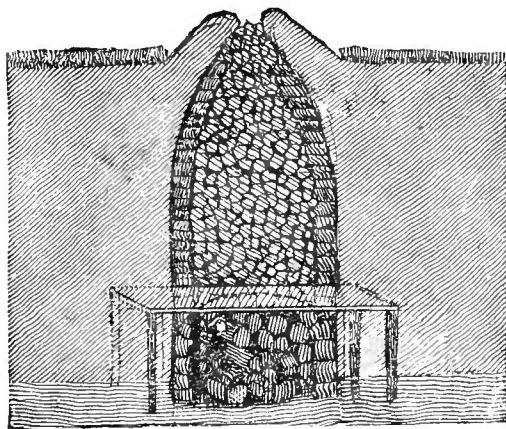
Fig. 190.—A LIME KILN.
