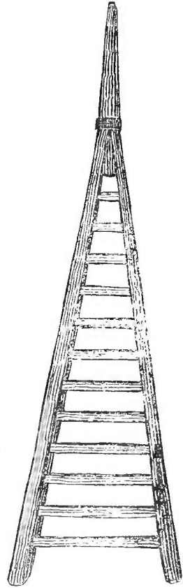
Fig. 213.—FRUIT LADDER.
