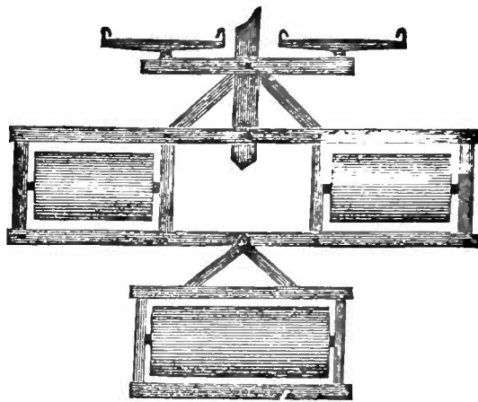
Fig. 47.—A TRIPLE LAND ROLLER.
