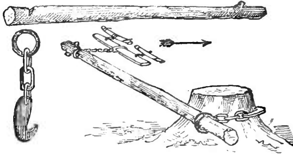
Fig. 176.—A SIMPLE STUMP-PULLER.
