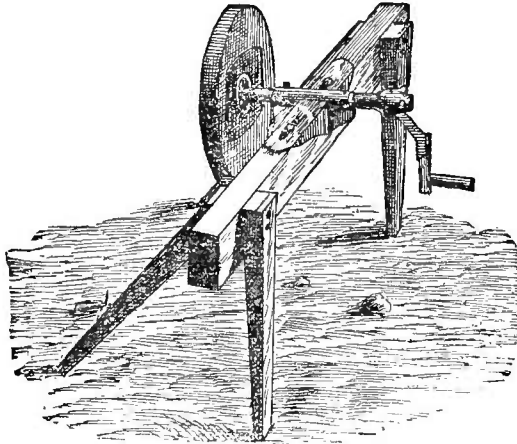
Fig. 71.—GRINDSTONE FRAME.
