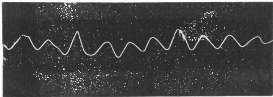
Fig. 8. — Courbe volumétrique d'un bras plongé dans de l'eau à 80.
